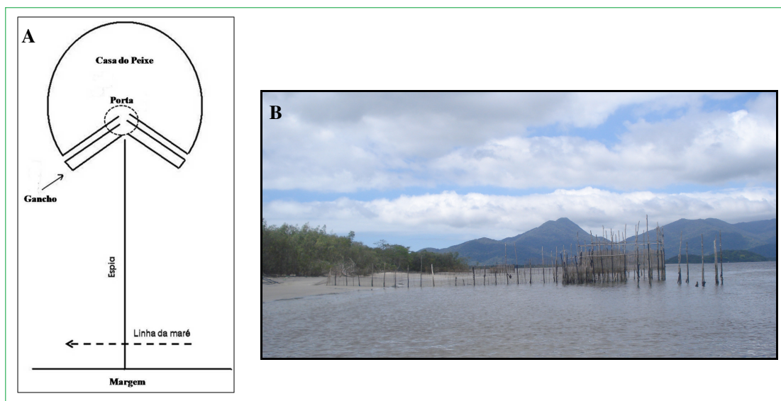
FIGURA 2: a) Desenho esquemático de um cerco-fixo; b) Cerco-fixo localizado na região da Ponta da Trincheira (Ilha Comprida) (Foto: Projeto Tartarugas / IPeC).
