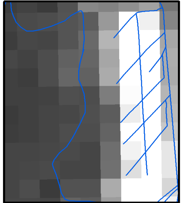
NDVI
